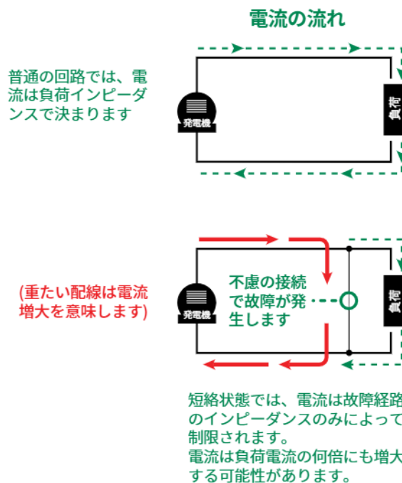
図 16 – 正常及び短絡における電流の流れ
