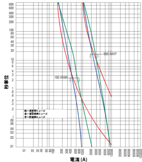
図5 - ヒューズ 3 種類の平均溶断時間比較
