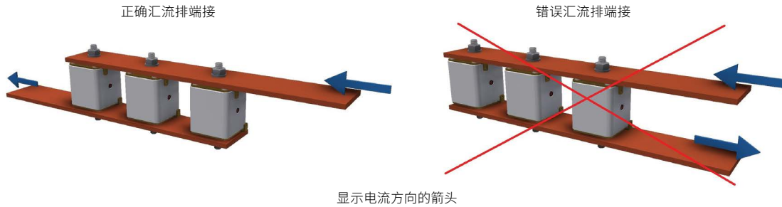
图 37: 并联两个或以上高速熔断器
