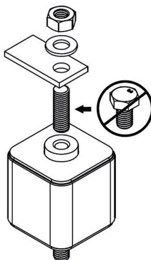
图 38: 推荐的熔断器端接方式
