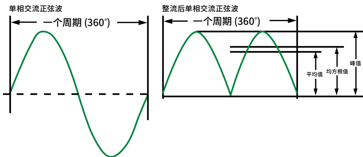
图 25: 均方根电流图示
