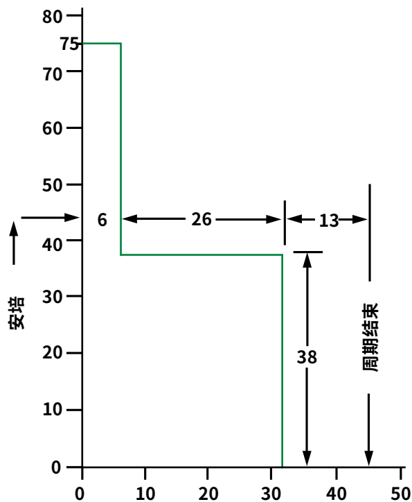
图 28: 循环电流说明
