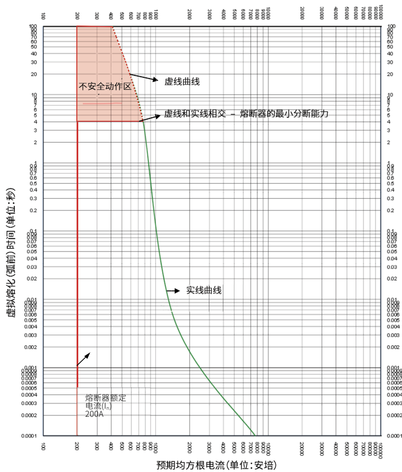
熔断器的不安全操作区
