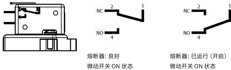
图 41: 带 NO-NC 触点的 MS 微动开关电路
