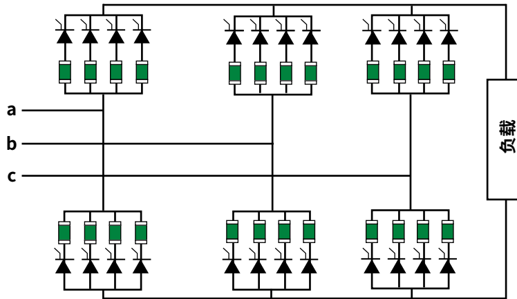
图 29: 整流器电路中的多并联连接
