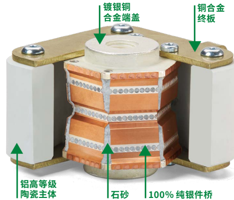
图 10b: 正方形主体样式熔断器
