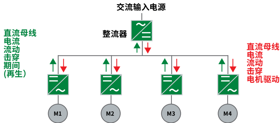
图 36: 直流母线配置
