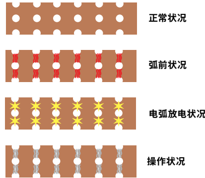
图 12: 操作期间熔断器元件的变化
