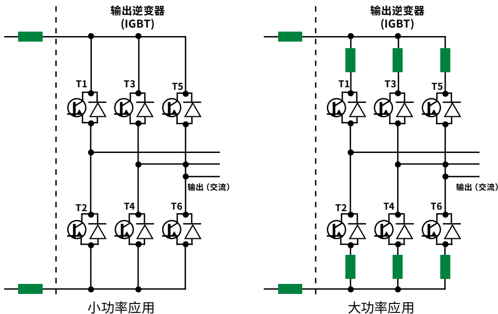
图 35: 高速熔断器在逆变器中的位置
