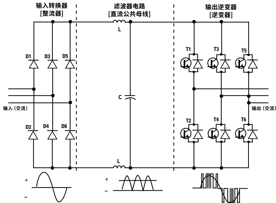
图 33: 典型三相功率转换器电路
