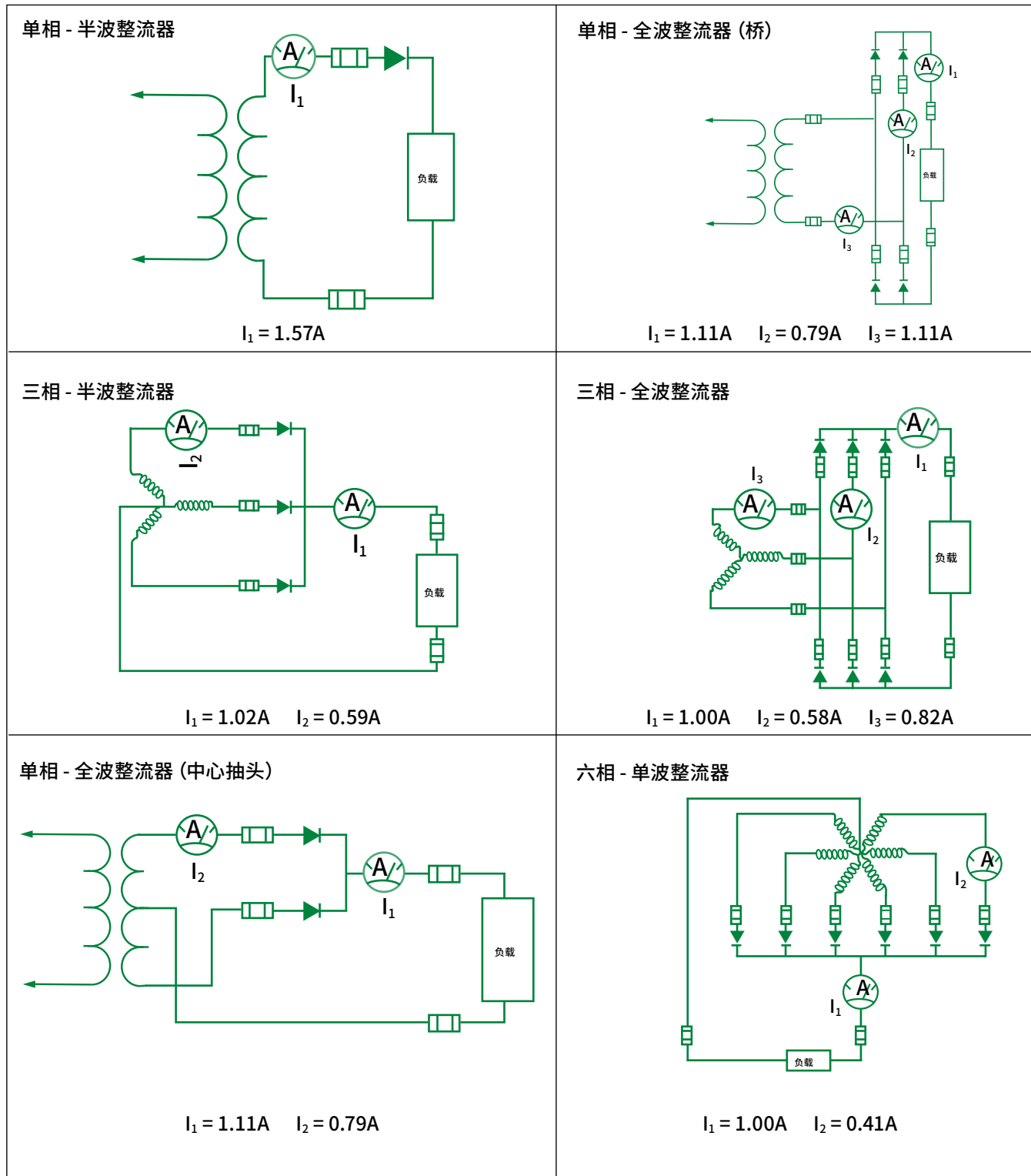
图 26: 典型整流器电路和电路中高速熔断器的位置
