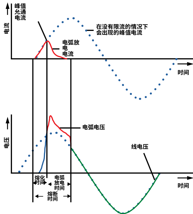
图 13: 熔断器操作期间的电流和电压性能
