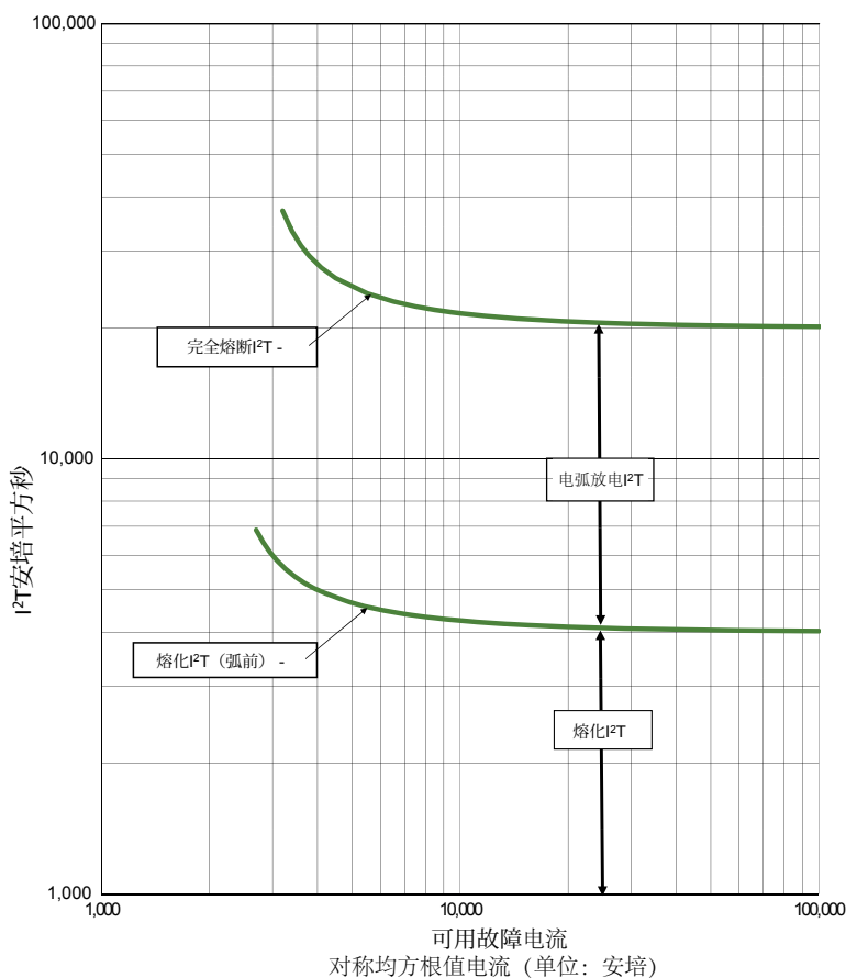
图 19: I^2t 特性曲线
