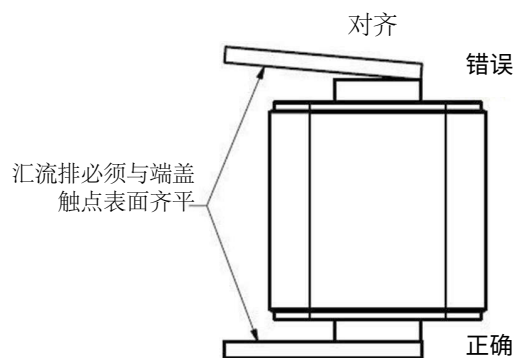
图 40 推荐的熔断器安装对齐
