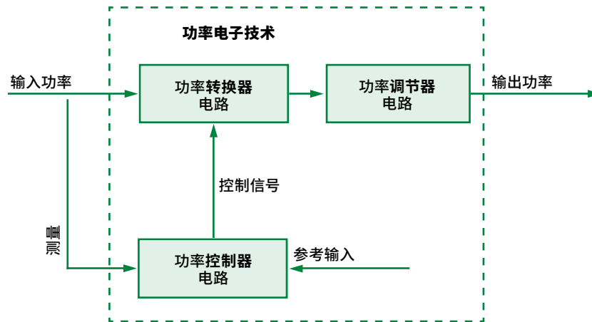
图 1: 功率电子系统框图
