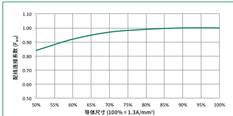
图 31: 配线连接系数 ( F_{WR} ) 曲线
