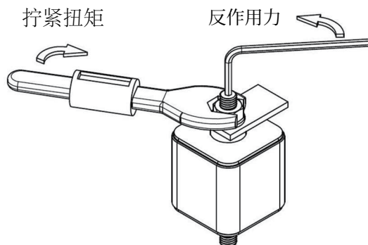
图 39: 推荐的建立连接的方式
