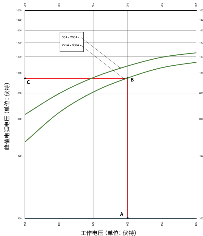
图 21: Littelfuse 高速熔断器的峰值电弧电压曲线
