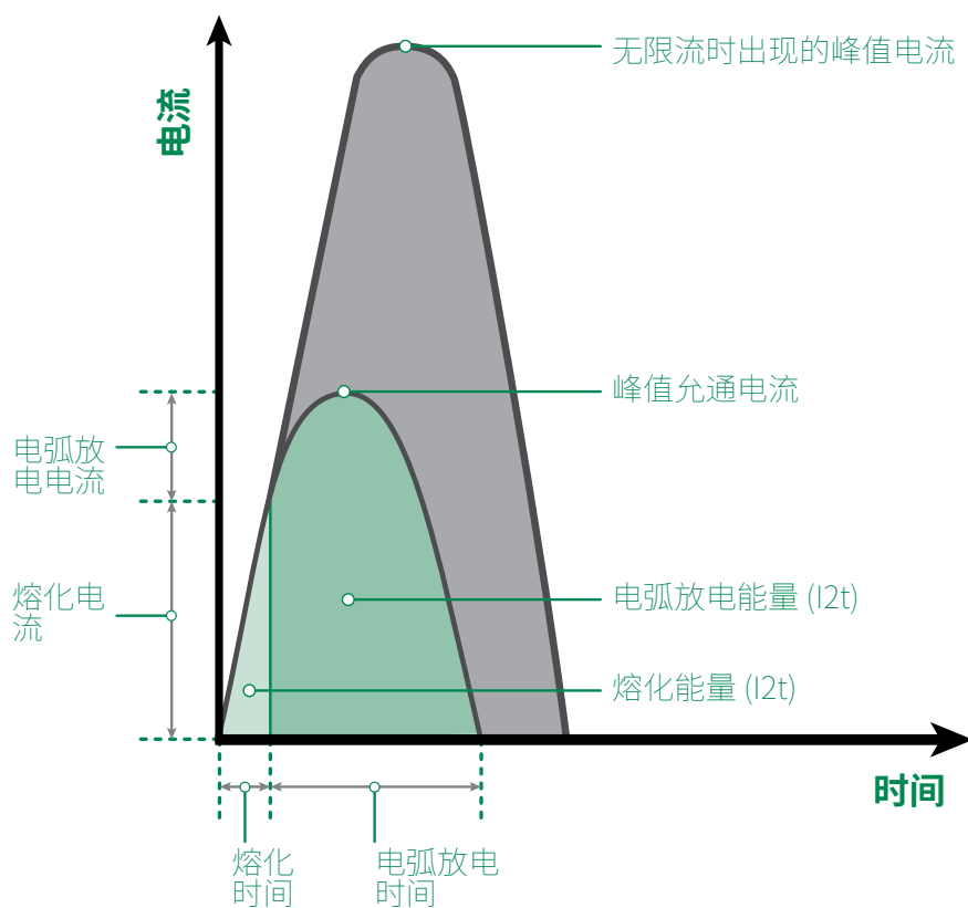
图 16: 熔断器的限流效应
